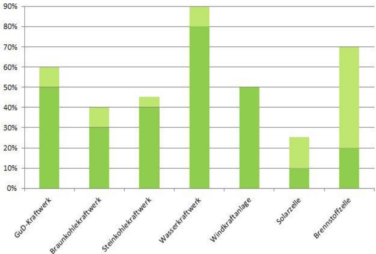
Abbildung 2: Wirkungsgrade verschiedener Strom erzeugender Kraftwerke
