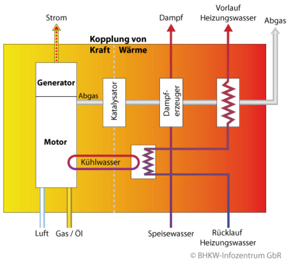
Abbildung 17: Beispiel einer KWK-Anlage
